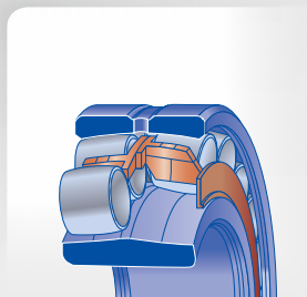
Umhüllungsprofil zur Führung der Wälzkörper
