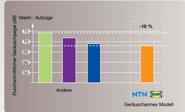
Histogramm des Geräuschpegels für eine Anwendung bei Aufzugsantrieben.
