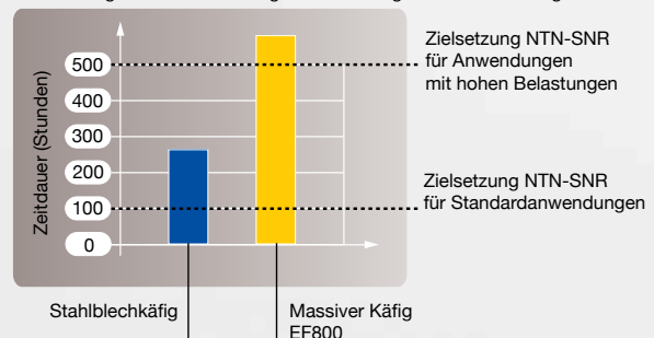
Versuchsergebnis aus dem Vergleich des Käfigs EA mit dem Käfig EF800
