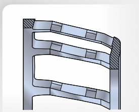
Optimierter Käfig für Serien 240xx und 241xx
