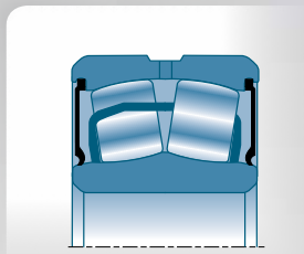
Modell ULTAGE EA abgedichtet
