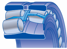
4 Führungs- und Halteleisten der Wälzkörper pro Baueinheit
