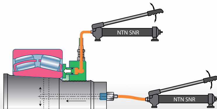
Gleichzeitige Verwendung von Hydraulikmutter und Einspritzung des Ölfilms
