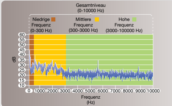
Beispiel des Akustikspektrums, das bei einem in Rotation versetzten Pendelrollenlager gemessen wurde.
