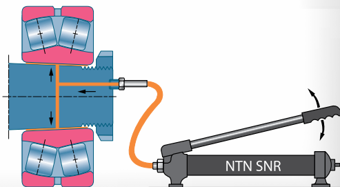
Prinzip der hydraulischen Demontage, weil Ölspritzkanäle vorhanden
